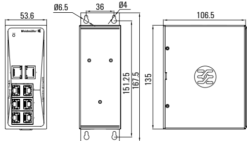
壁挂安装尺寸图
