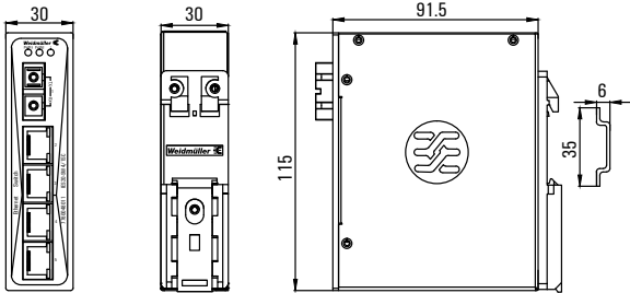
卡轨安装尺寸图
