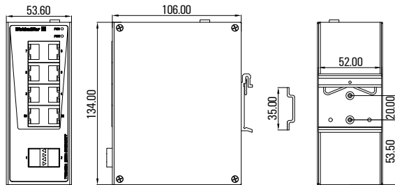
安装尺寸图
