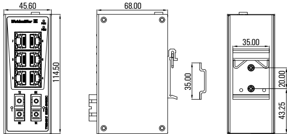
安装尺寸图
