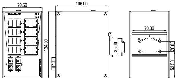
安装尺寸图
