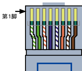
T568A线序
