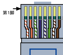
T568B线序
